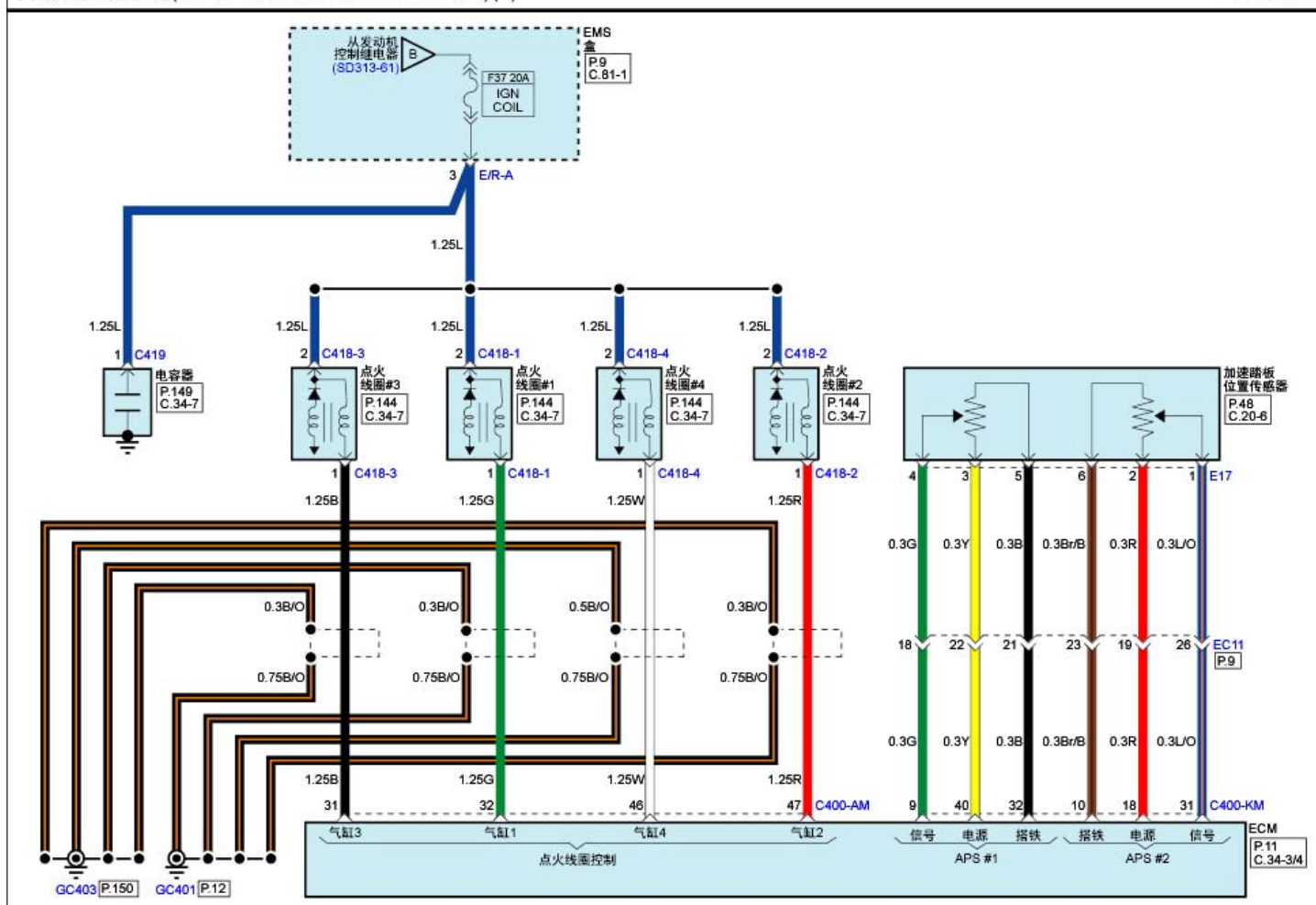
发动机控制系统(G4FJ: GAMMA 1.6L T-GDI M/T)(6)
